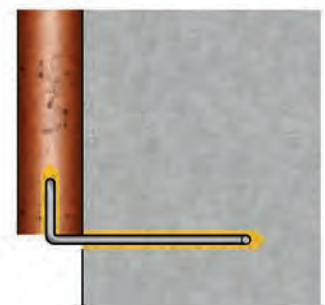
INSTALACIÓN DE LA GAS EN LAS PIEZAS FINALES DE LA CUBIERTA GAS INSTALLING IN THE FINAL PIECES OF THE COVER INSTALLATION DU GAS DANS LES DERNIÈRES PIÈCES DU COUVERTURE
